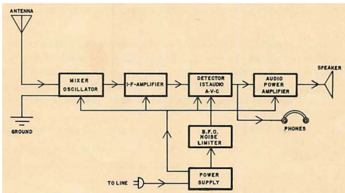
מקלט S-38 : מרשם מלבנים מקור: חוברת היצרן
