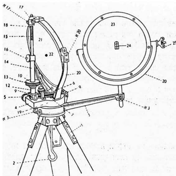
הליוגרף עם מראת משנה
