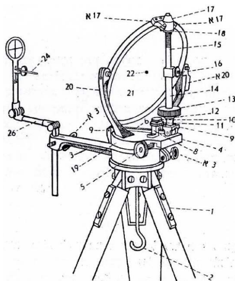
הליוגרף עם קנה כיוון מתקפל
