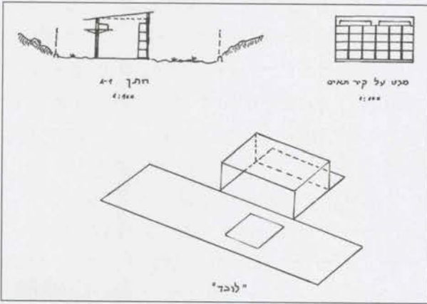
תכנית ה'לובד', מיועד לקליטת יונה בהגיעה לפתח השובך
